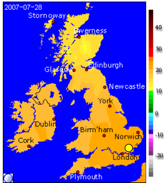
Forecast Max Temperature (°C) Sat 28 Jul
